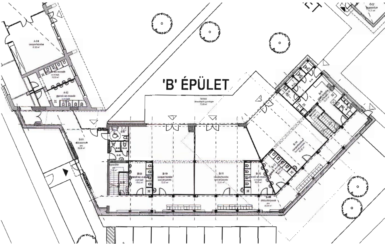
FÖLDSZINTI ALAPRAJZ
