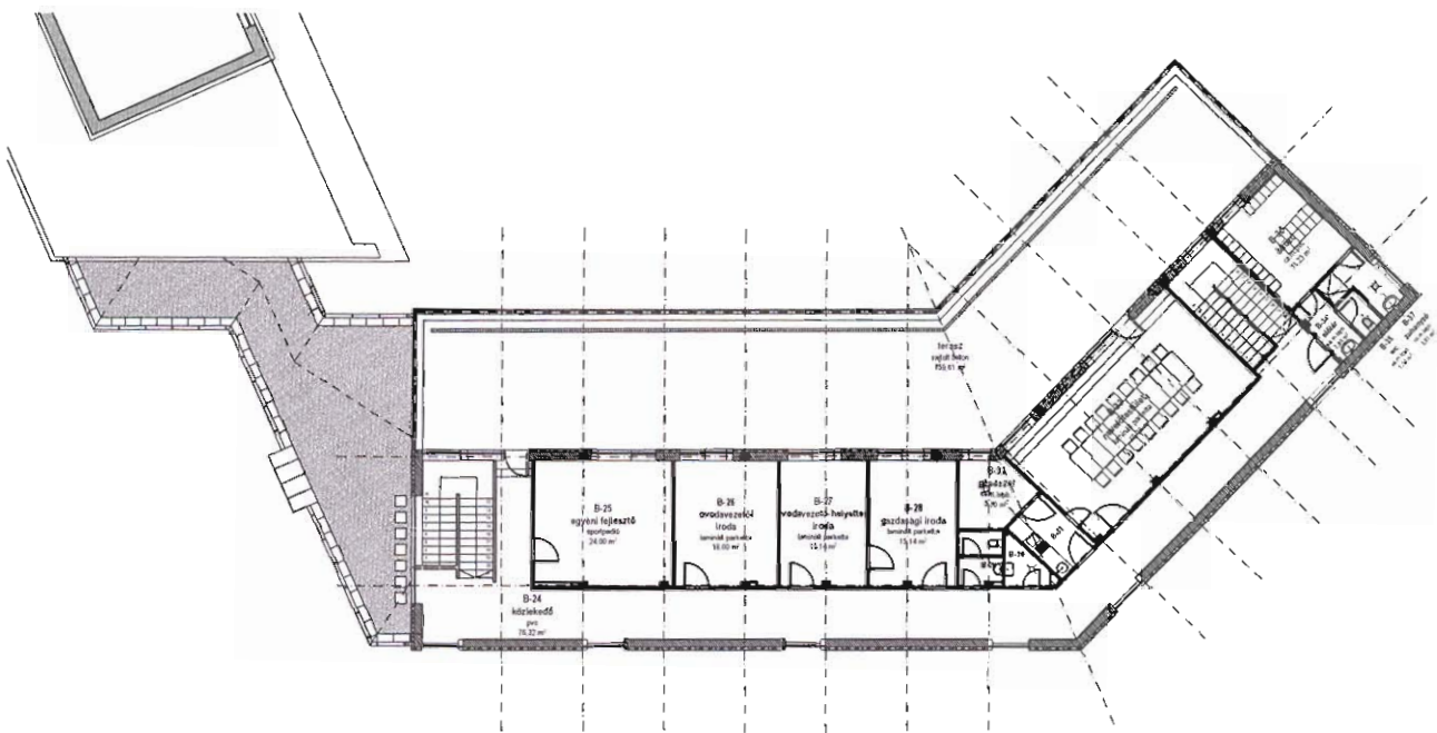
EMELETI ALAPRAJZ
